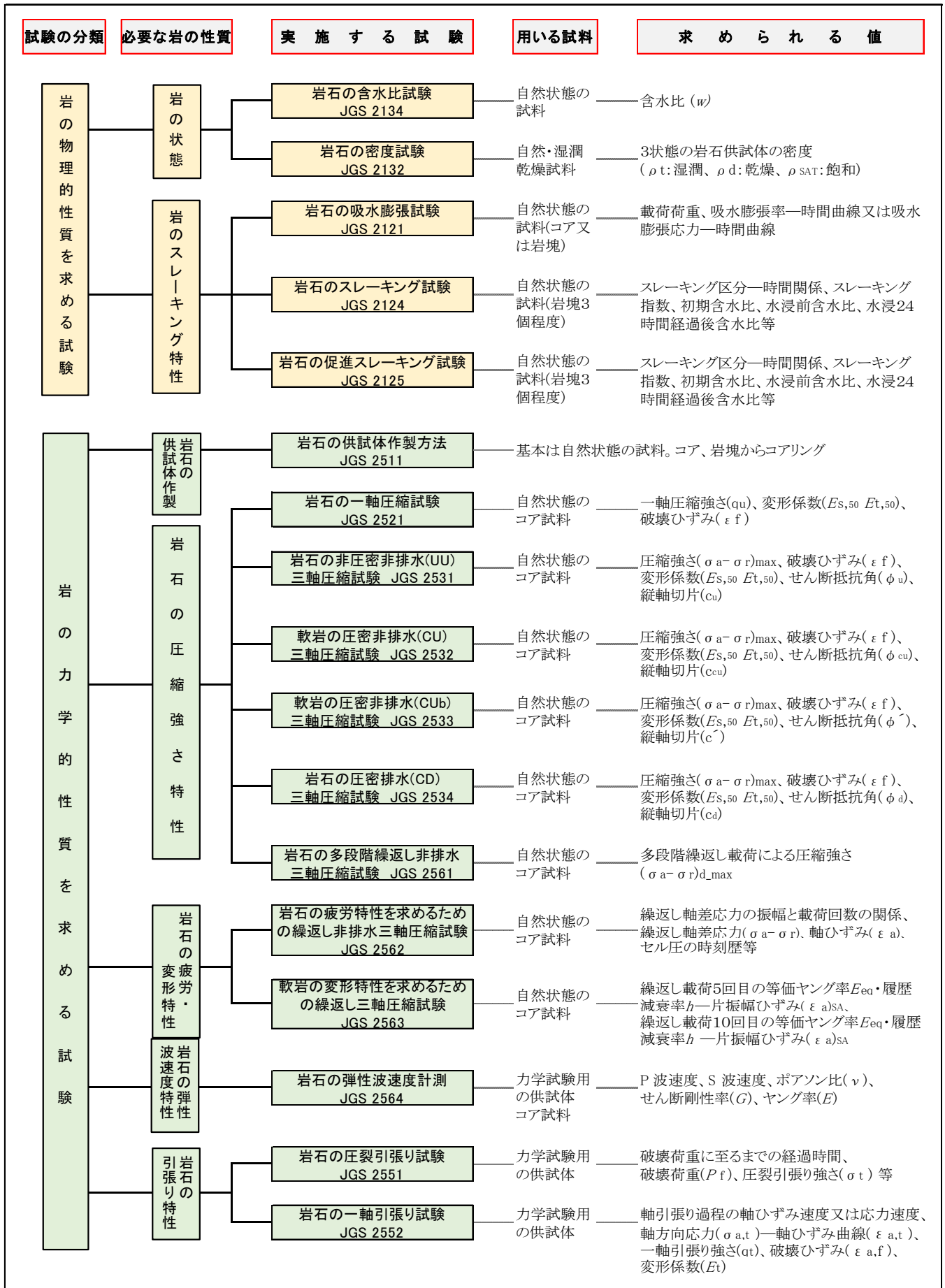
図-4.2 岩石試験の目的及び試験の種別等 (4に基づき新たに作成)
