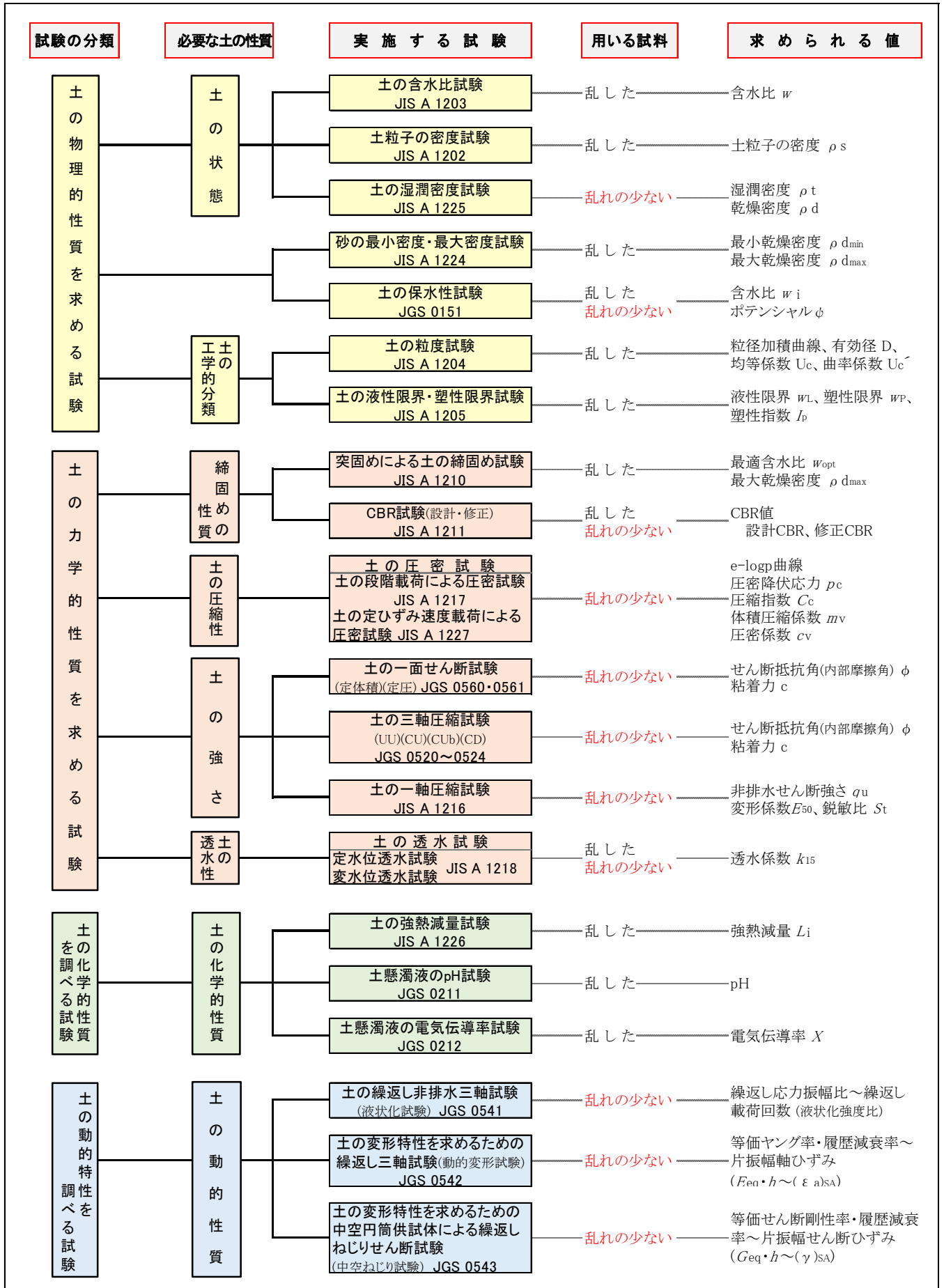
図-4.1 地盤材料試験(土質試験)の目的及び試験の種別等(3-部加筆)
